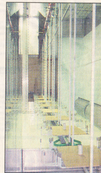
Ny lackeringsanläggning. Om bara några veckor tas den här nya lackeringsanläggning i bruk. På bandet rullar olika möbeldelar genom anläggningen där två robotar sköter lackeringen.
